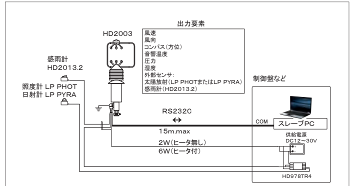
RS232Cシリアル通信のシステム図
