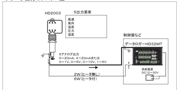
アナログ出力のシステム図
