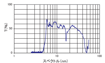
Fig.2 シリコンウインドウの透過率
