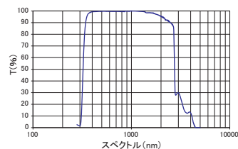
Fig.1 全天日射計の相対スペクトル応答
