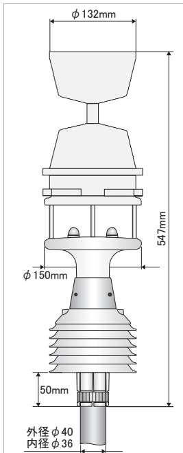
HD52.3DT147 風速、風向、雨量、温度、 相対湿度、大気圧
