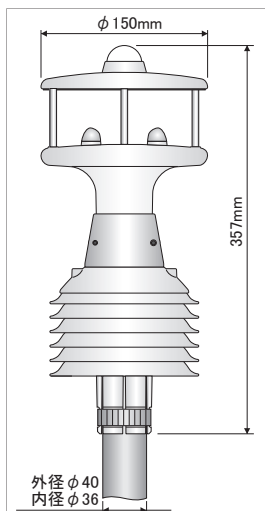
HD52.3DP17 風速、風向、日射量、温度、 相対湿度
