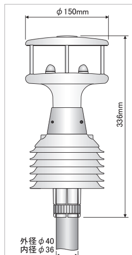
HD52.3D17 風速、風向、温度、相対湿度
