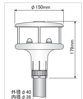
HD52.3D 風速、風向
