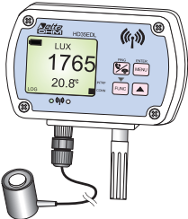
照度および UVセンサ
