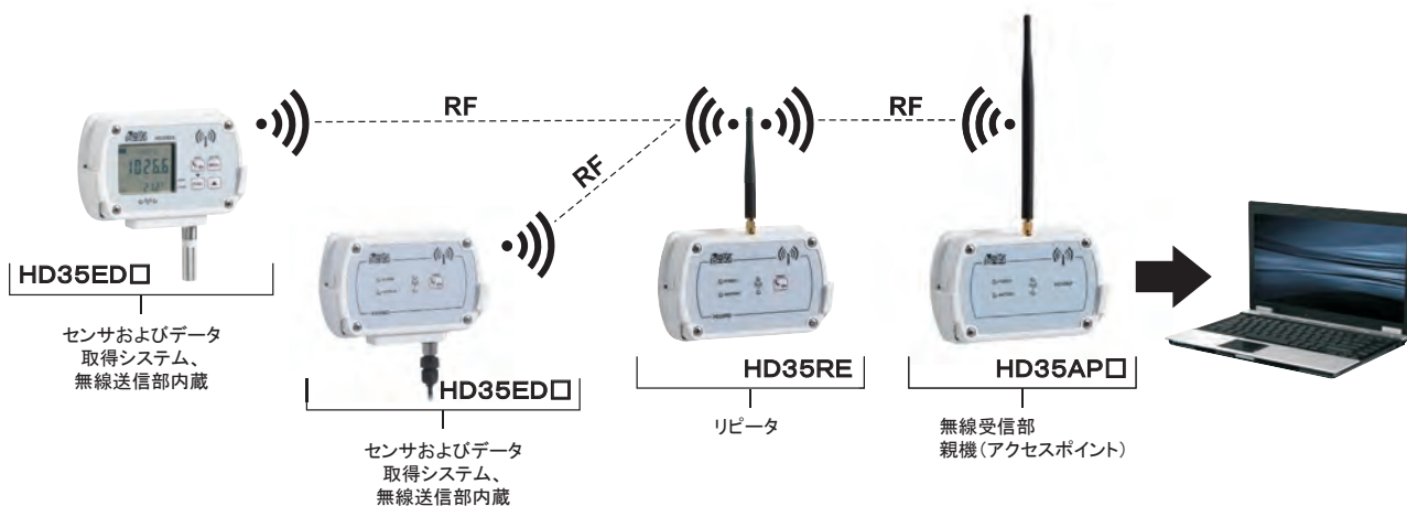
ワイヤレスデータロギングシステム、リピータ使用
