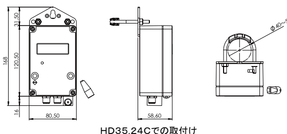
HD35.24Cでの取付け
